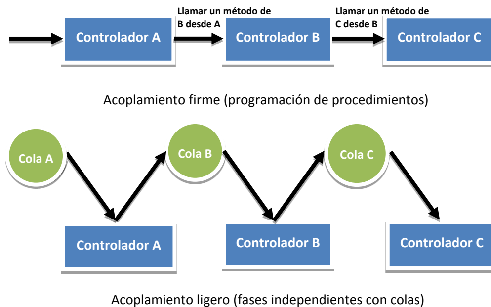
Ilustración 3: desacople de componentes mediante la utilización de Colas
