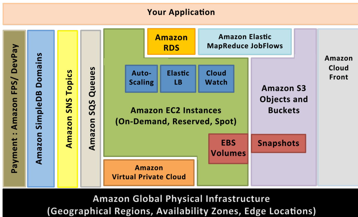
Ilustración 1: Amazon Web Services
