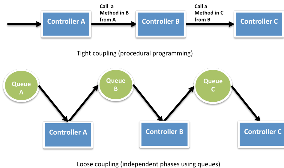
Ilustración 3: desacople de componentes mediante la utilización de Colas
