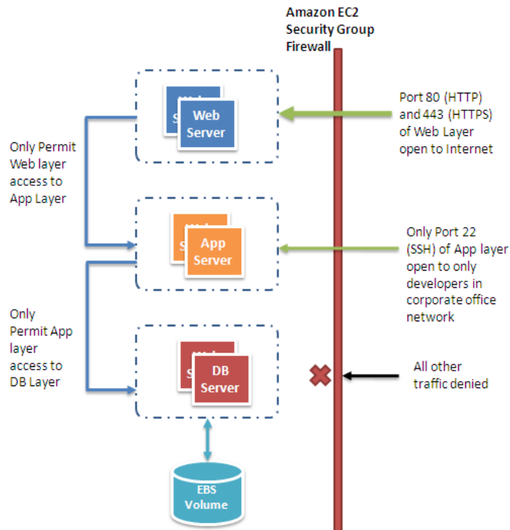
Ilustración 4: Proteger su aplicación web mediante grupos de seguridad de Amazon EC2
